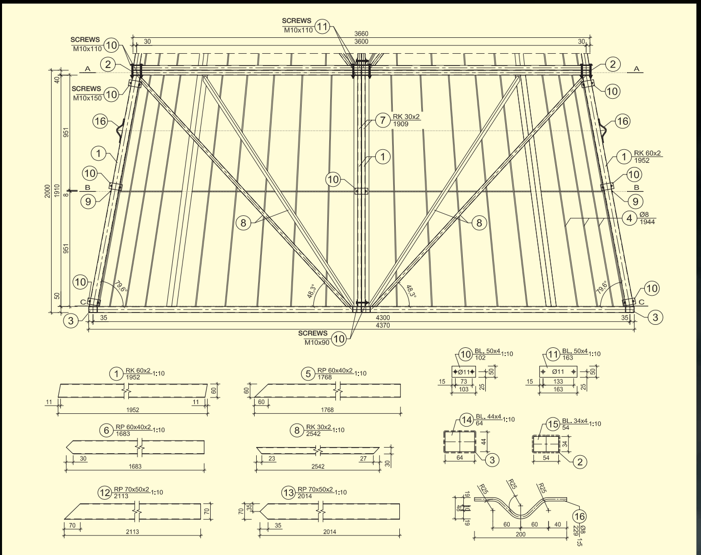
Detailed description of elements of a selected segment (12-14) / Szczegółowy opis elementów wybranego segmentu (12-14)
