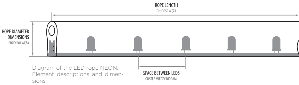
Schemat węża NEON LED. Opisy elementów i wymiarowań.
