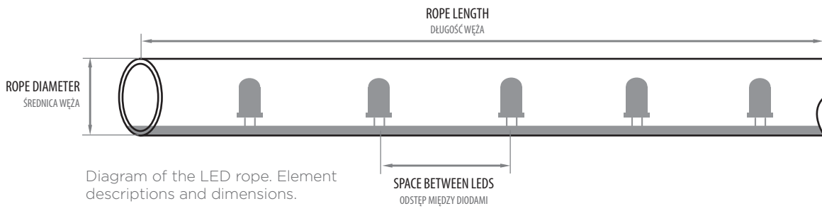
Schemat węża LED. Opisy elementów i wymiarowań.
