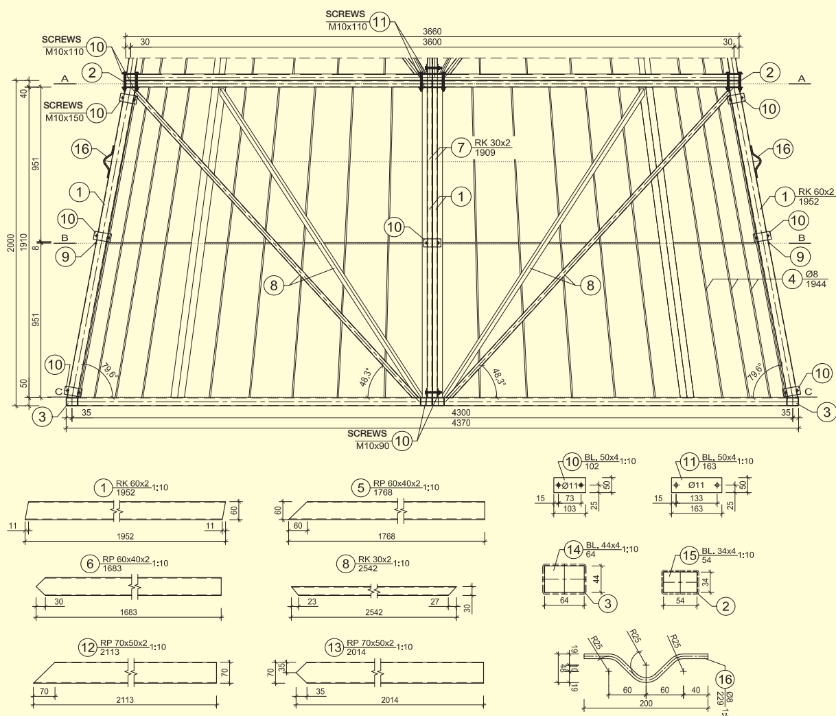
Detailed description of elements of a selected segment (12-14) / Szczegółowy opis elementów wybranego segmentu (12-14)
